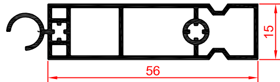
PU 203 Cierre portamanija
