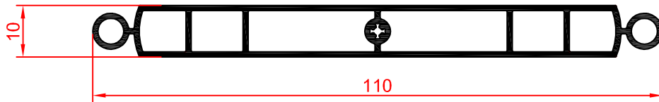
PU 203 Cierre portamanija
