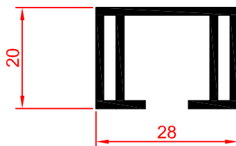
PU 206 Bisagra Hembra
