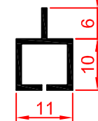
PC 435 Perfil para colgado 10 x 11 mm
